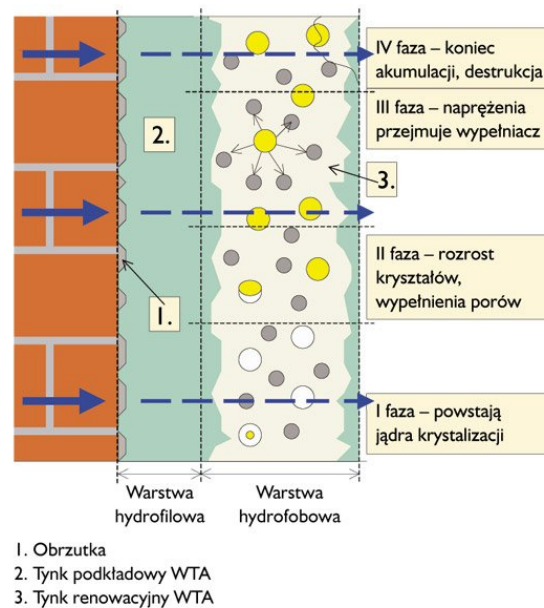
Rys. 10. Budowa i zasada funkcjonowania tynków renowacyjnych WTA.
