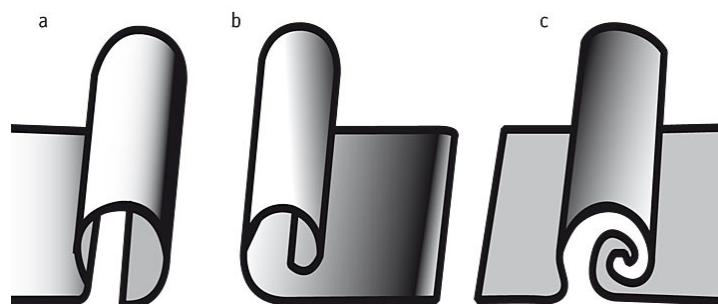
Rąbek leżący: a) pojedynczy b) podwójny
