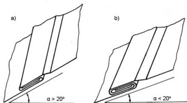
Rąbek leżący: a) pojedynczy b) podwójny
