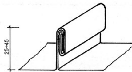
Rąbek stojący podwójny
