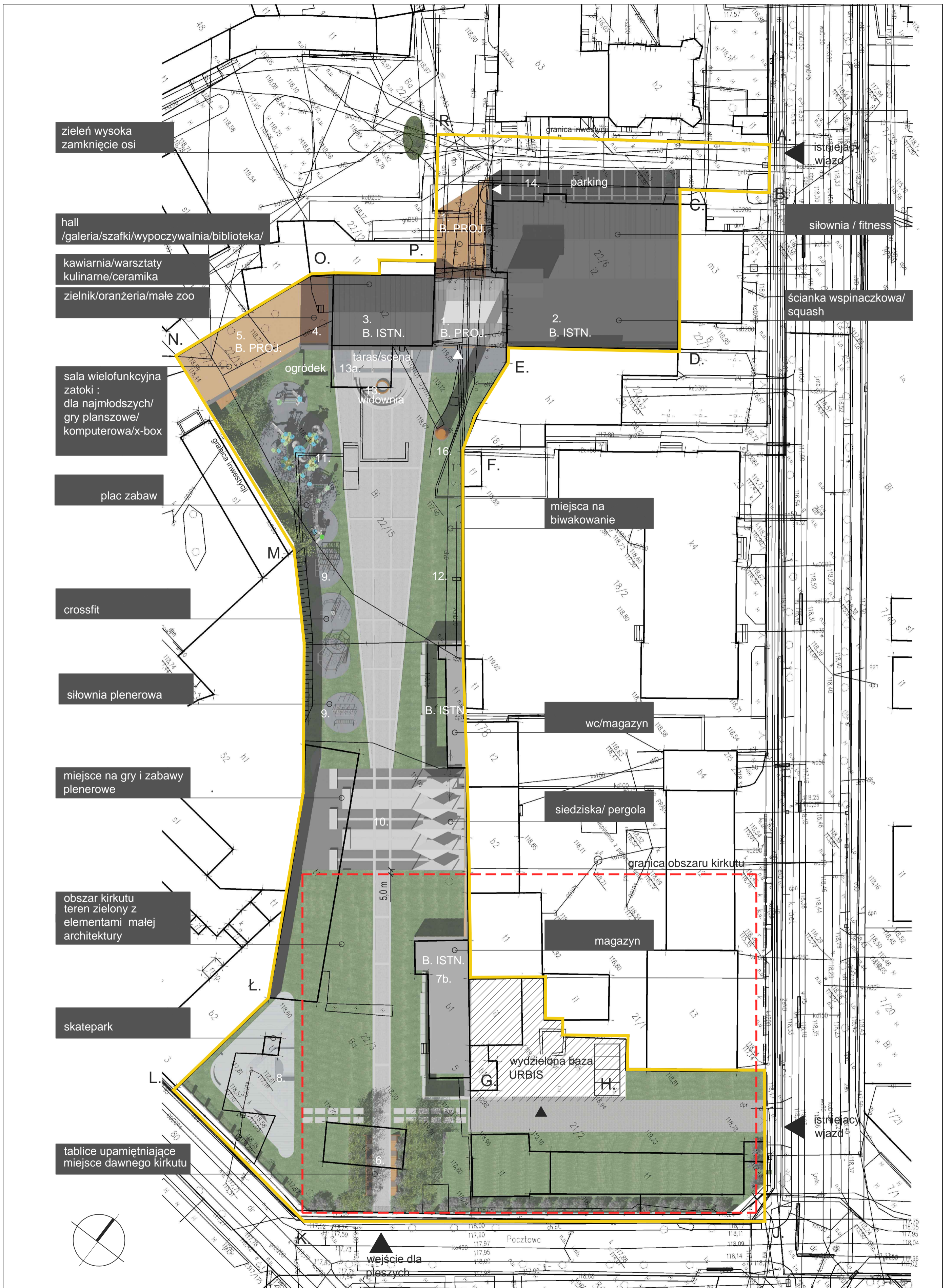
PLAN ZAGOSPODAROWANIA TERENU 1:500
