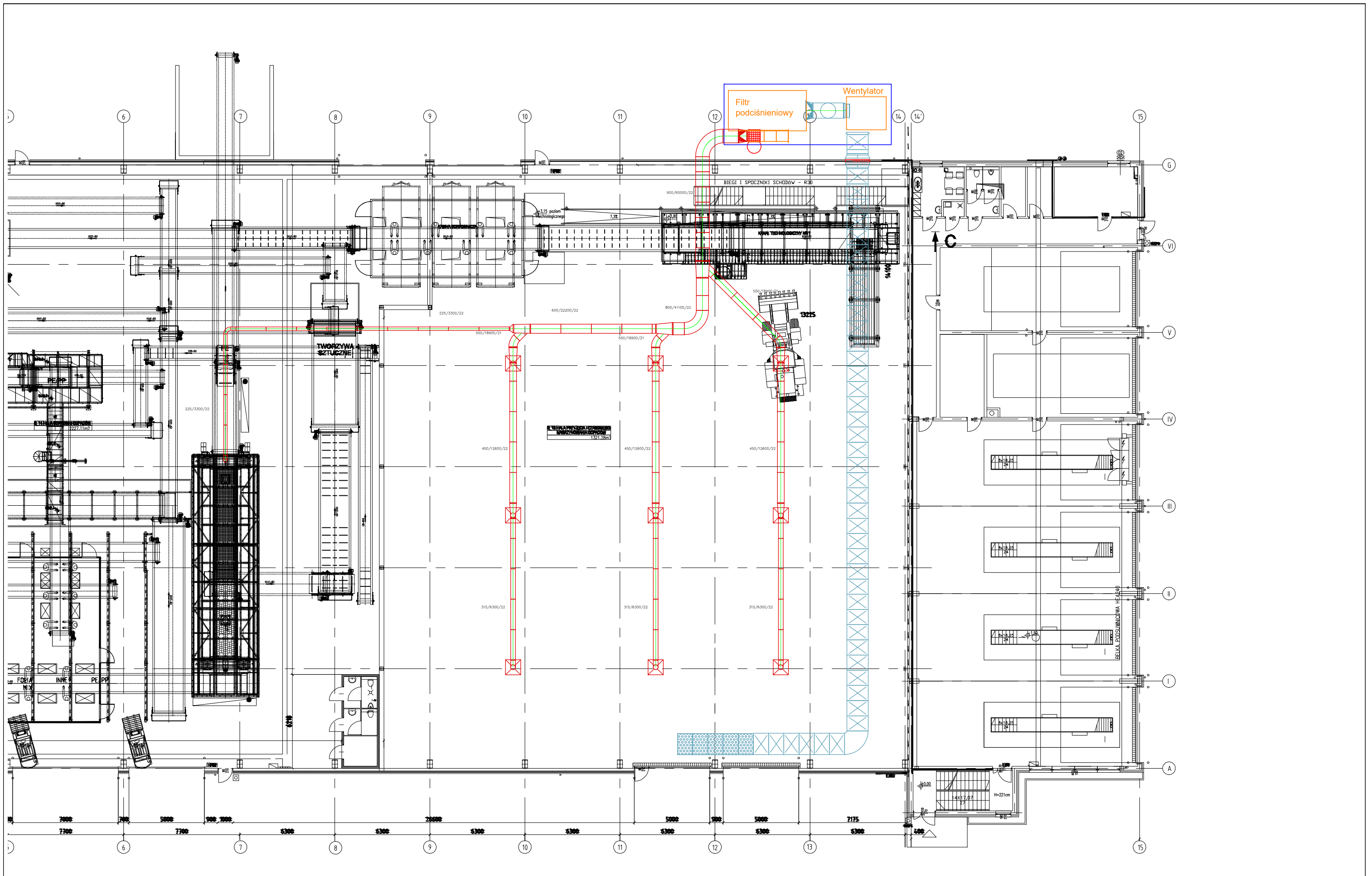
Rys. 2 - rzut hali sortowni z instalacją odpylania - Wariant I
